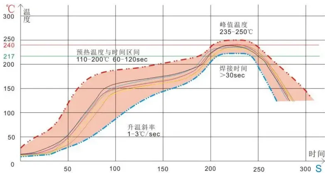
图 4 焊接炉温曲线
