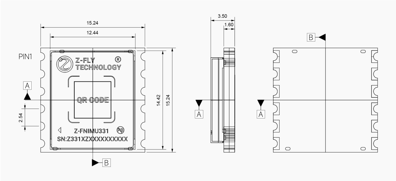
图2 推荐焊盘尺寸图（单位mm）
