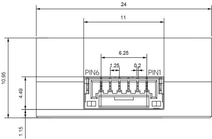
图2 接口尺寸图（单位mm）
