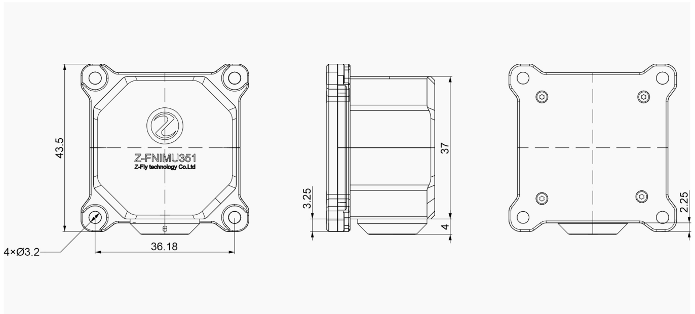
图2 接口尺寸图（单位mm）
